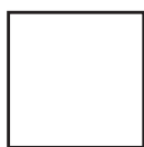
Segi empat beraturan (persegi)
