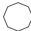
Segi delapan beraturan
