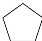
Segi lima beraturan
